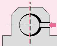
従来のサイドロック 芯ズレしてしまう
